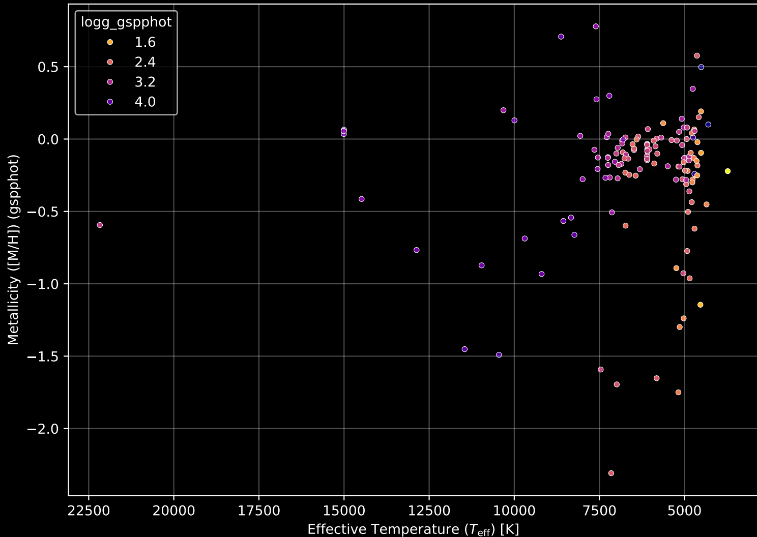
APOGEE DR17 Field: [263-03] Stellar Population Parameters (n= 139)
